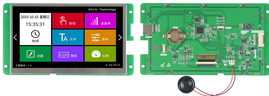
图 1-3 7.0 寸无触摸参考图
