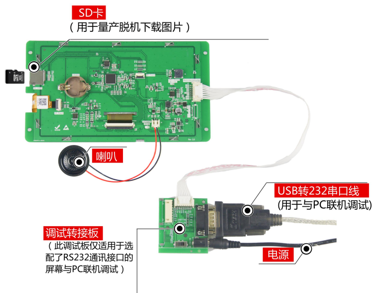
图 1-5 调试工具图
