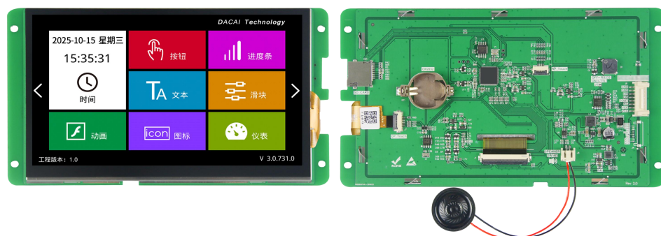
图 1-2 7.0 寸电容触摸参考图
