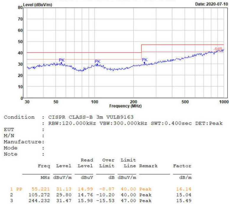
图 4-5 RE 测试水平方向
