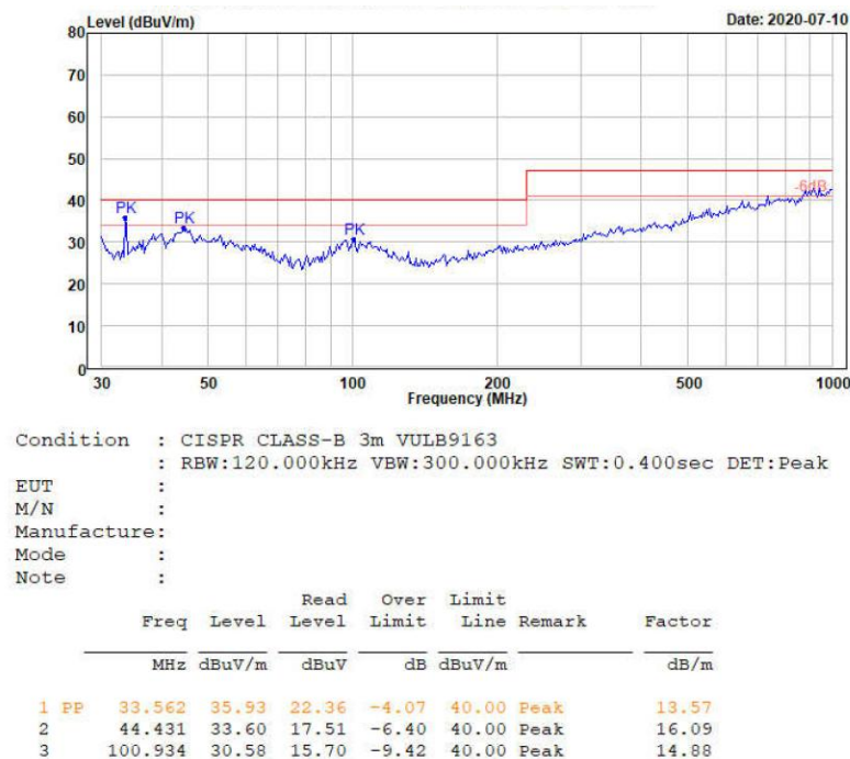
图 4-6 RE 测试垂直方向
